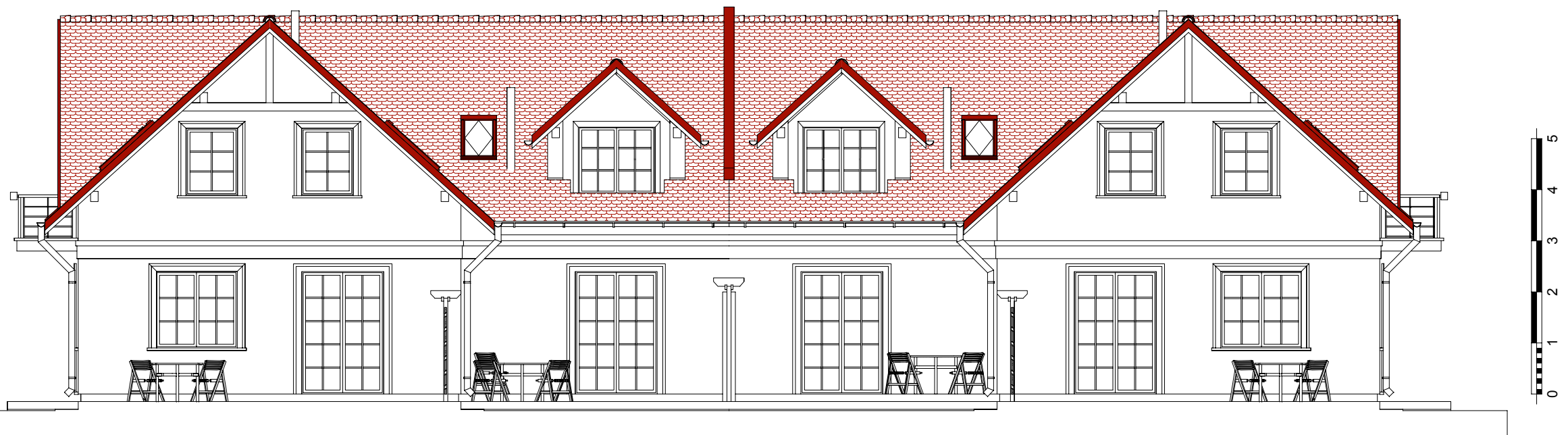
0 1 2 3 4 5 Pohled zahradní 1:100
